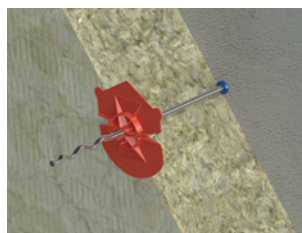
UNI-slagspouwanker Ø4 mm met kraagplug art. 34118 + UNI-clip rood art. 34130
