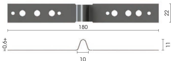
Lijmbouwmuuranker dilaterend
