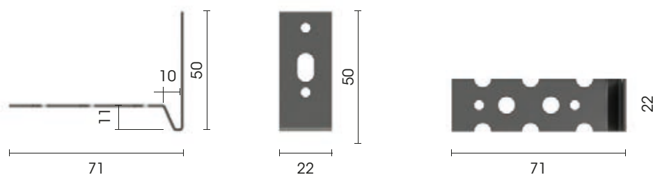
Lijmbouwmuuranker dilaterend
