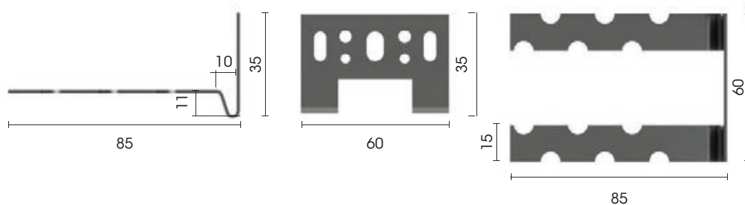
Wandanker dilaterend
