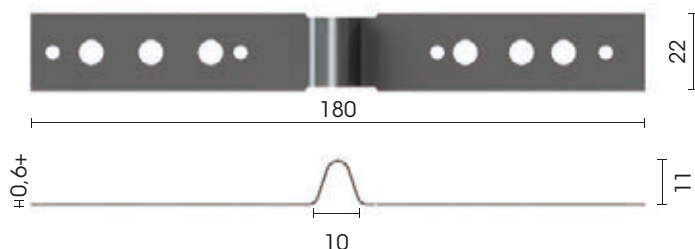
Lijmbouwmuuranker dilaterend
