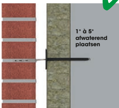
figuur 1, richtlijnen spouwanker verwerking
