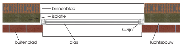
Schematische weergave montage tegen het BUITENspouwblad
