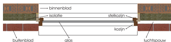
Schematische weergave montage tegen het BINNENspouwblad
